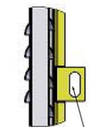
DETTAGLIO B SCALA 1:4
